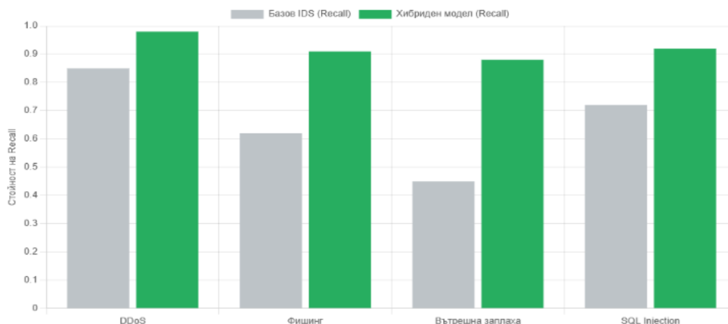
Фиг. 3. Сравнителен анализ: Традиционен IDS vs. Предложен хибриден модел.
