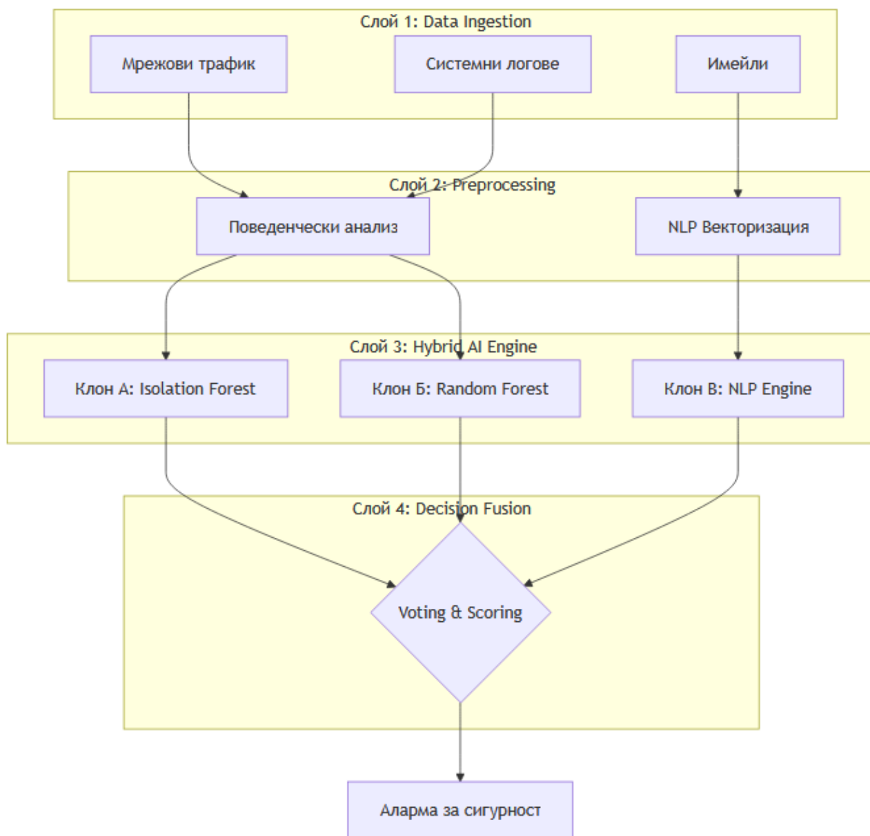
Фиг. 1. Обработка на данни от събиране до финално решение.
